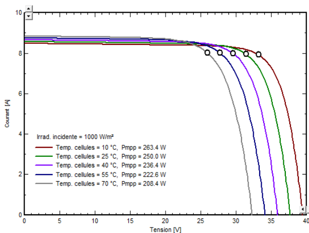
Module PV: NR Sol, NRS 60P250
