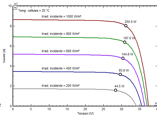
Module PV: NR Sol, NRS 60P250
